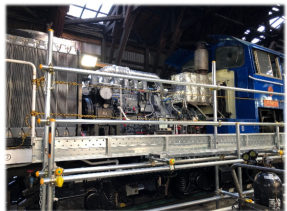
DD5653 号機関換装工事
